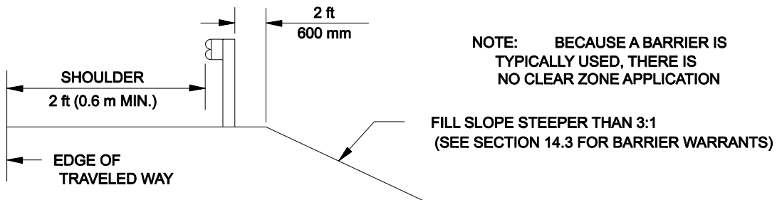
CRITICAL PARALLEL SLOPE (d)
